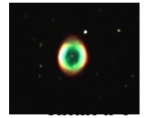
La matière dans l'Univers.
